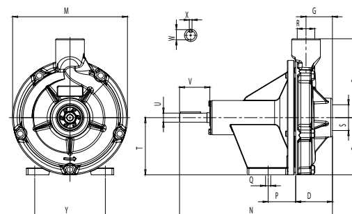
DIMENSÕES EM MILÍMETROS (mm) 60 Hz
