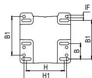
VISTA INFERIOR PÉ DO MOTOR
