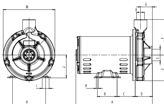
DIMENSÕES EM MILÍMETROS (mm) 60 Hz
