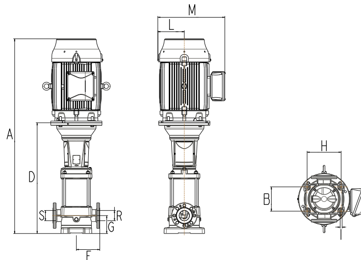
DIMENSÕES EM MILÍMETROS (mm) - 60 Hz
