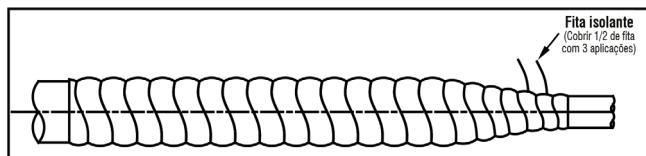
Figura 7: Terceira isolamento (fita isolante)
