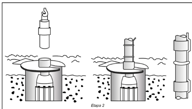
Figura 9: Esquema com sugestão de montagem
