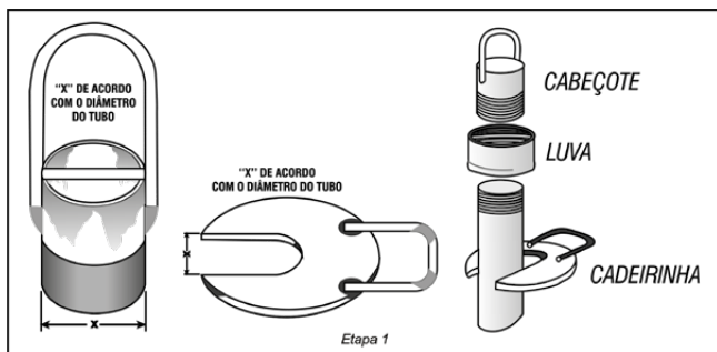
Figura 8: Esquema com sugestão de montagem
