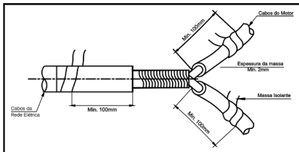
Figura 5: Primeira isolamento (massa isolante)
