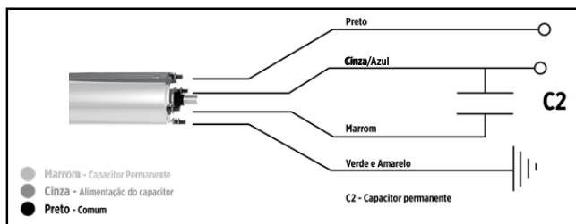
Figura 13: Esquema de ligação série MS4 OL.
