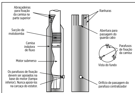
Figura 4: Camisa indutora de fluxo
