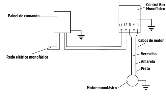
Figura 15: Esquema de ligação motores monofásicos 3 fios.
