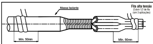
Figura 6: Segunda isolamento (fita de alta tensão)
