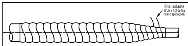
Figura 7: Terceira isolamento (fita isolante)
