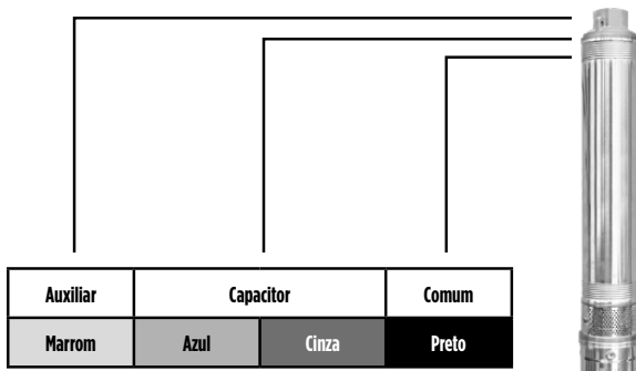
Figura 12: Esquema de ligação série SUB 2,5 e SUB 3.
