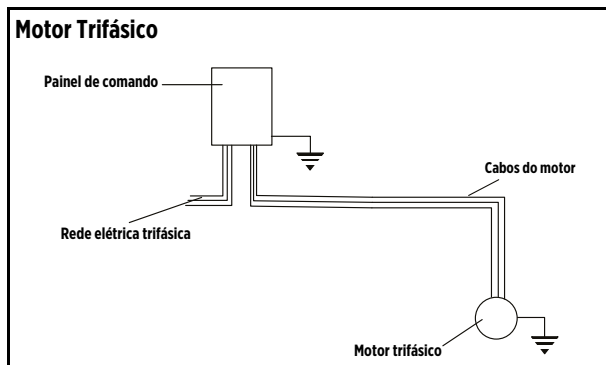
Figura 16: Esquema de ligação motores trifásicos.
