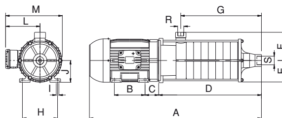
DIMENSÕES EM MILÍMETROS (mm) - 60 Hz
