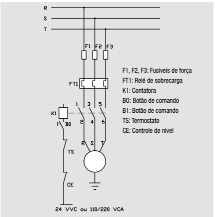
Figura 9 - Diagrama trifásico com contator
