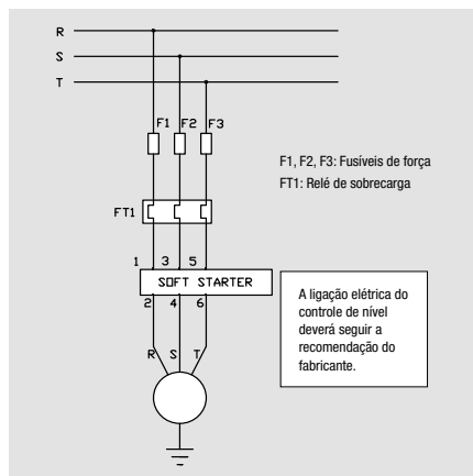
Figura 10 - Diagrama trifásico com soft starter até 2 cv
