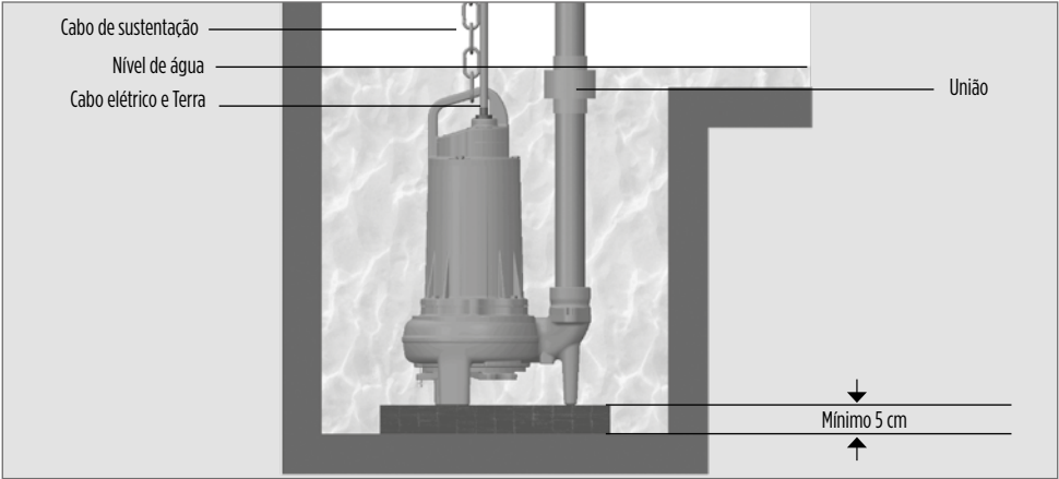
Figura 4 – Esquema de instalação da motobomba com sistema de acoplamento direto
