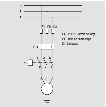
Figura 8 - Diagrama trifásico até 2 cv
