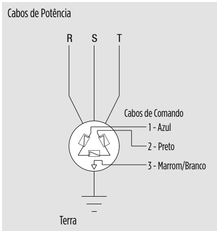
Figura 7 - Diagrama do motor
