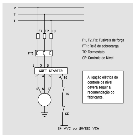
Figura 11 - Diagrama com soft starter a partir de 3 cv
