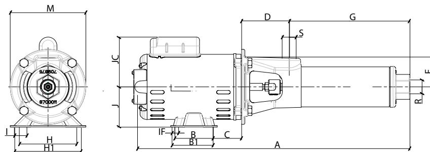
DIMENSÕES EM MILÍMETROS (mm) - 60 Hz
