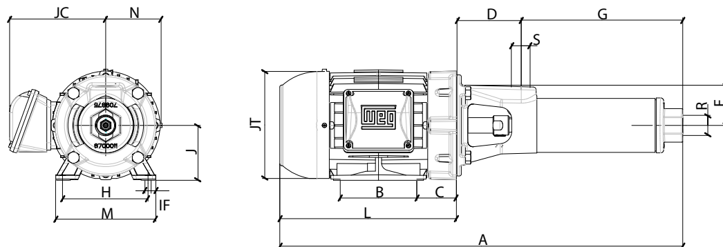
DIMENSÕES EM MILÍMETROS (mm) - 60 Hz BT4 (Motor IP-55)
