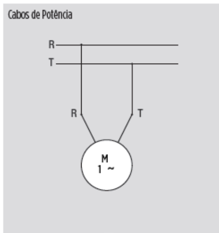
Figura 6 - Diagrama monofásico
