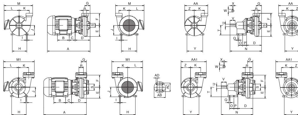
DIMENSÕES EM MILÍMETROS (mm) - 60 Hz
