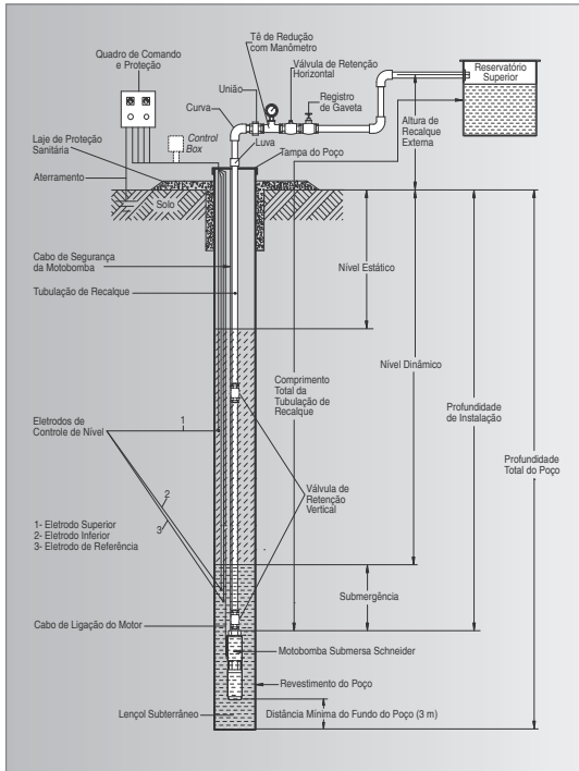
Figura 3: Esquema típico de instalação
