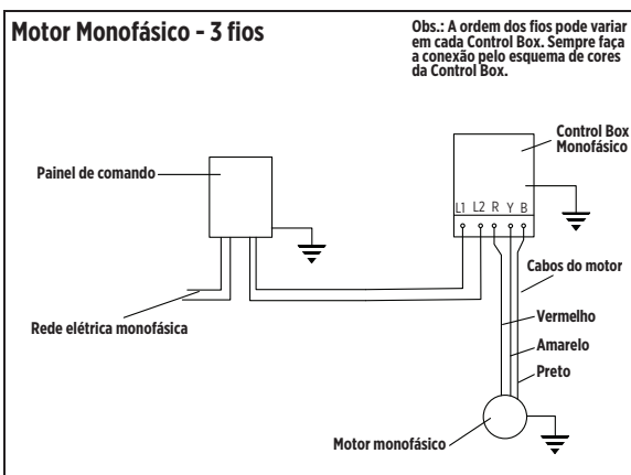
Figura 14: Esquema de ligação motores monofásicos 3 fios.
