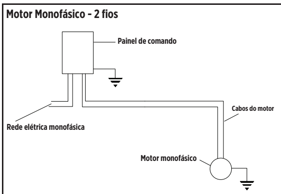
Figura 13: Esquema de ligação motores monofásicos 2 fios.
