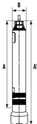
DIMENSÕES EM MILÍMETROS (mm) - 60 Hz
