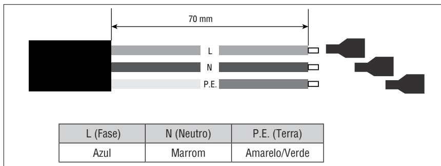
Figura 3B - Identificação dos cabos elétricos
