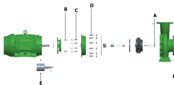
Figura 10 - Componentes de aperto
