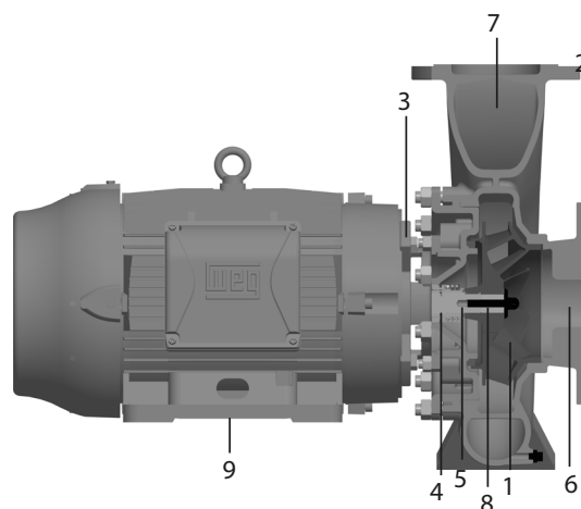
Figura 3 - Componentes
