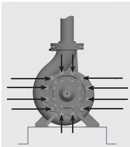
Figura 8 - Vista do intermediário ilustrando parafusos
