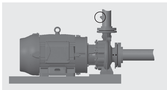
Figura 6 - Instalação bujão de escorva
