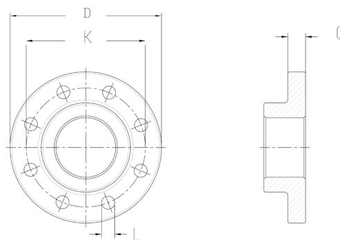
Figura 4 - Dimensional dos flanges
