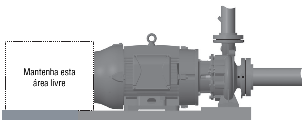
Figura 7 - Motobomba sem obstáculo para remoção de back pull-out
